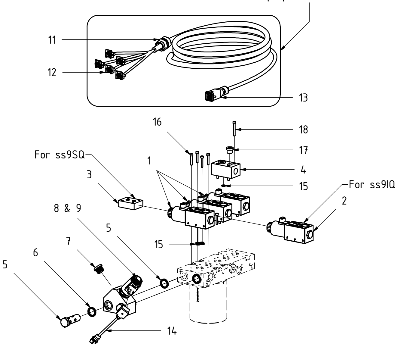
Assembly Cable ss9 Dump (pos. 10): 1006950
