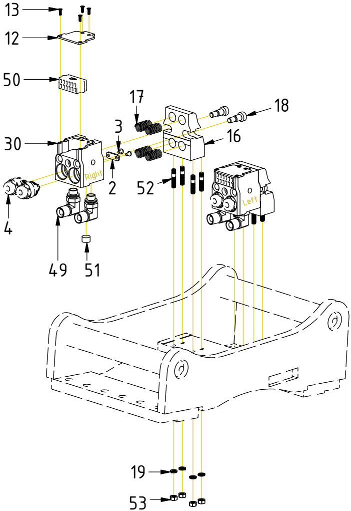
Top bracket QS45 Modular config.
