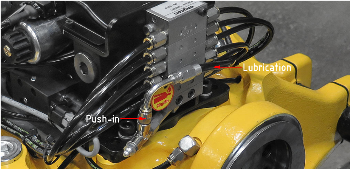
Lubrication
