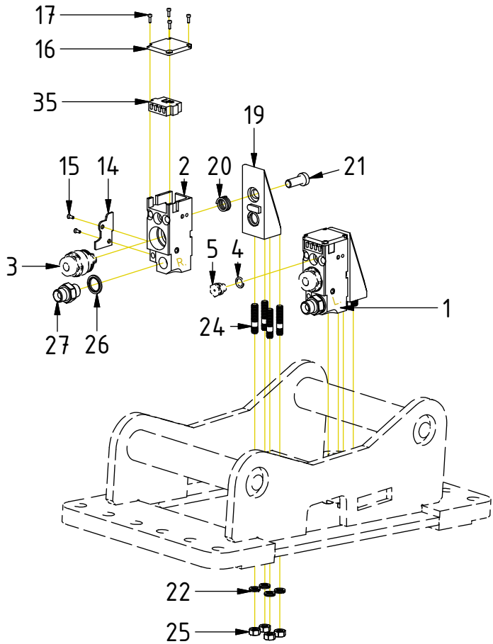
Top bracket QS40 Modular config.
